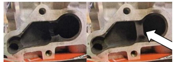
Figura 3 – Cabeça de motor original (à esquerda) e modificada com adição de material (à direita).
