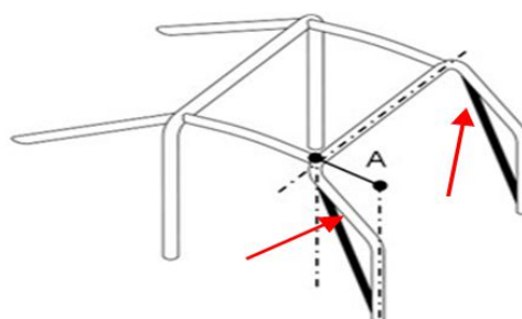
Figura 18 - Habitáculo / Reforço do montante do para-brisas
