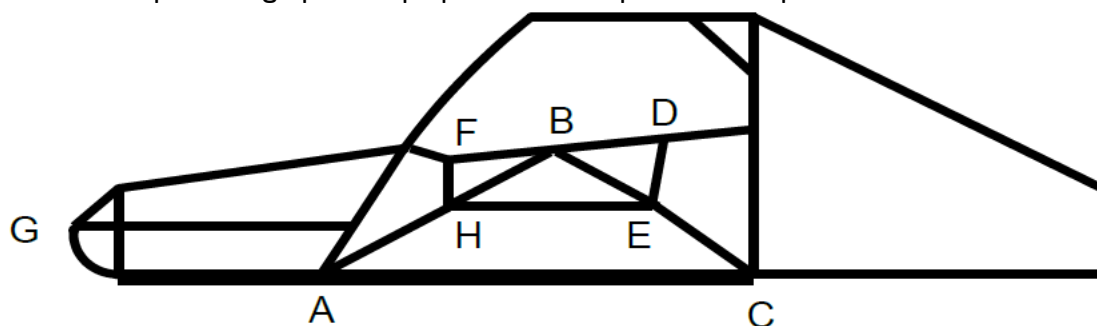
Figura 29 - Vista lateral do chassis
